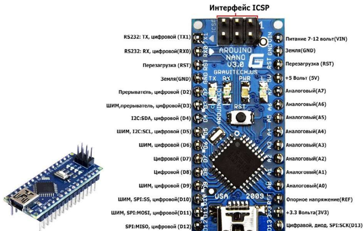
Рис. 120. Плата Arduino-нано
