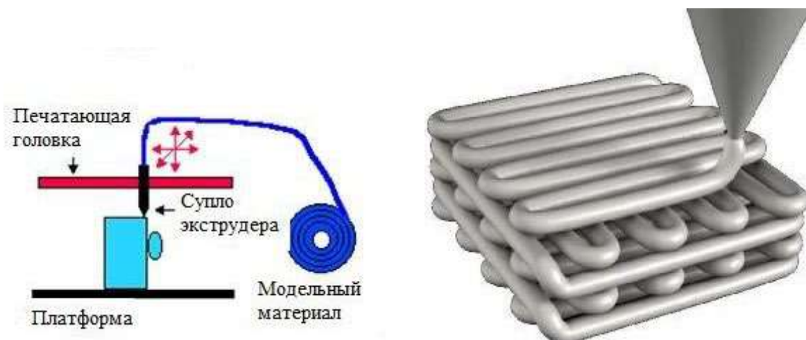
Рис. 56. Технология FDM
