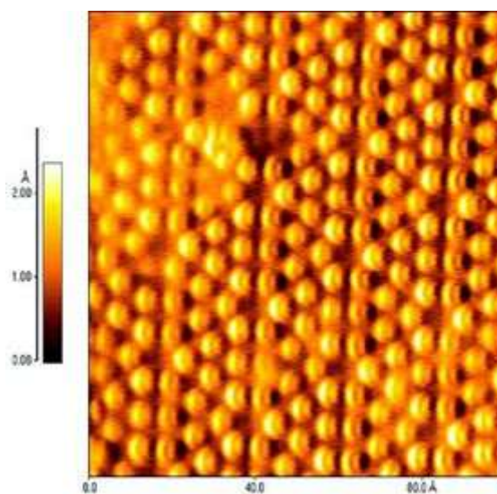
Рис. 109. Атом кремния
