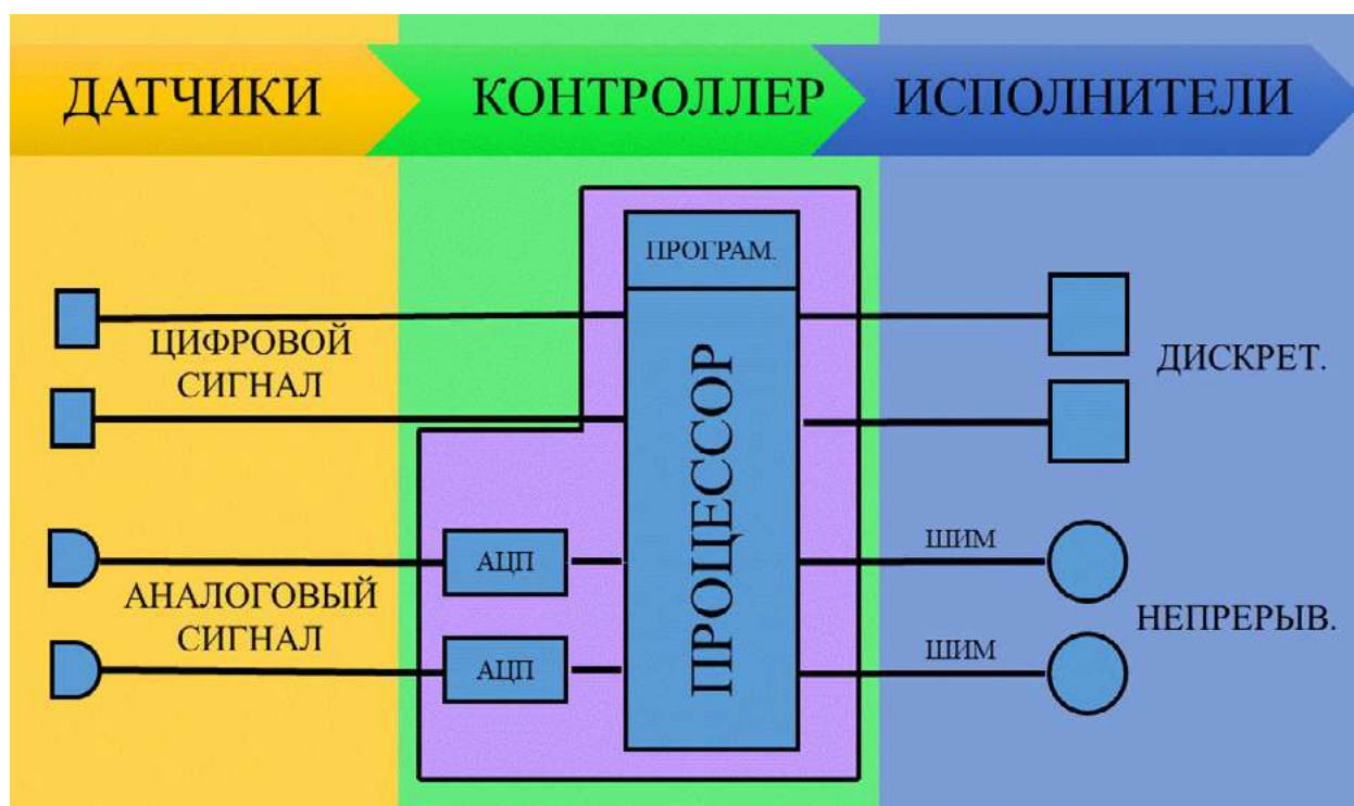
Рис. 119. Обработка сигнала
