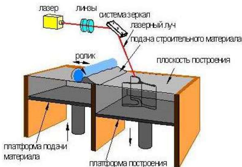
Рис. 54. Bed Deposition
