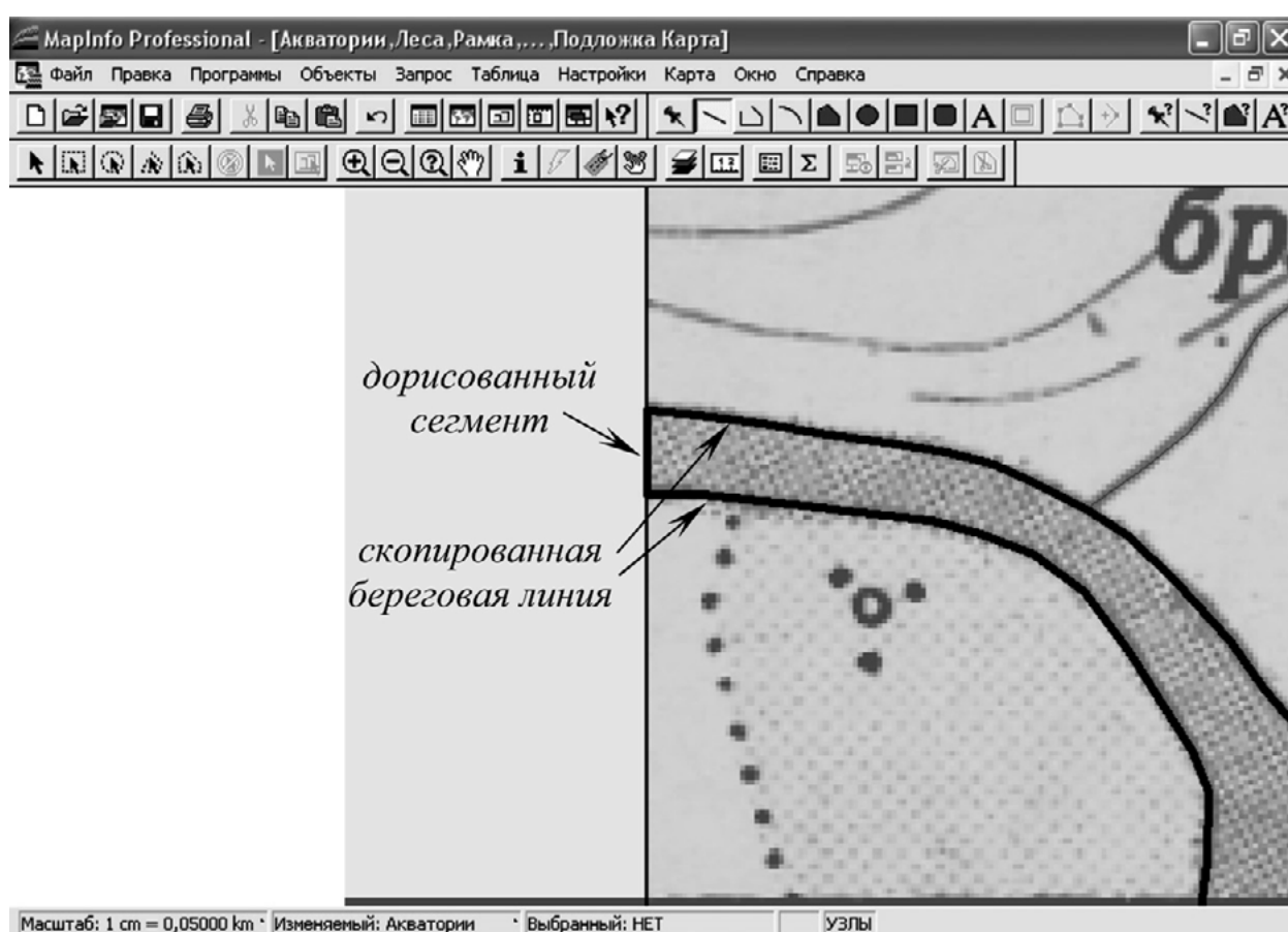
Рис. 84. Вид программы
